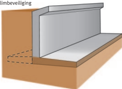
betonnen L-profiel
