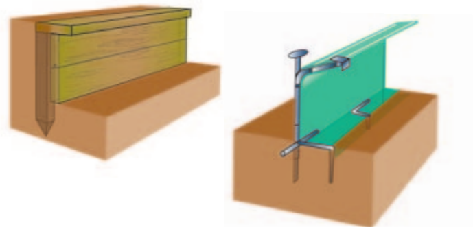
wand van hout of gerecycleerde kunststof • tijdelijk scherm van kunststofweefsel of -folie
