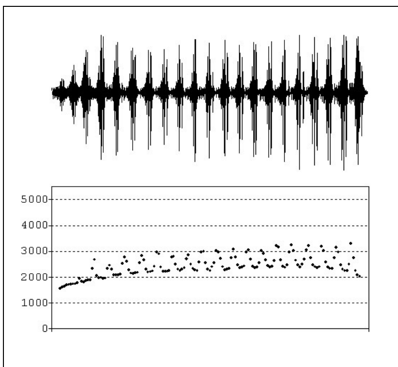
Fig. 7: Sonagram en frequentieverloop in functie van de tijd van een paringsroep van een mannetje Bastaardkikker ( P. kl. esculentus ) te Merelbeke (O.V.I.) ter vergelijking. De paringsroep duurt 0,917 sec. en bevat 21 pulsgroepen. Het gemiddeld frequentieverloop is 2428 Hz (min. 1559 Hz – max. 3285 Hz). Watertemperatuur 19-20° C.
